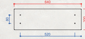
ثقوب التثبيت على الارضية مناسبة للتثبيت بوندد فولاذي 8م
