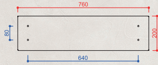
ثقوب التثبيت على الارضية مناسبة للتثبيت بوندد فولاذي 8م
